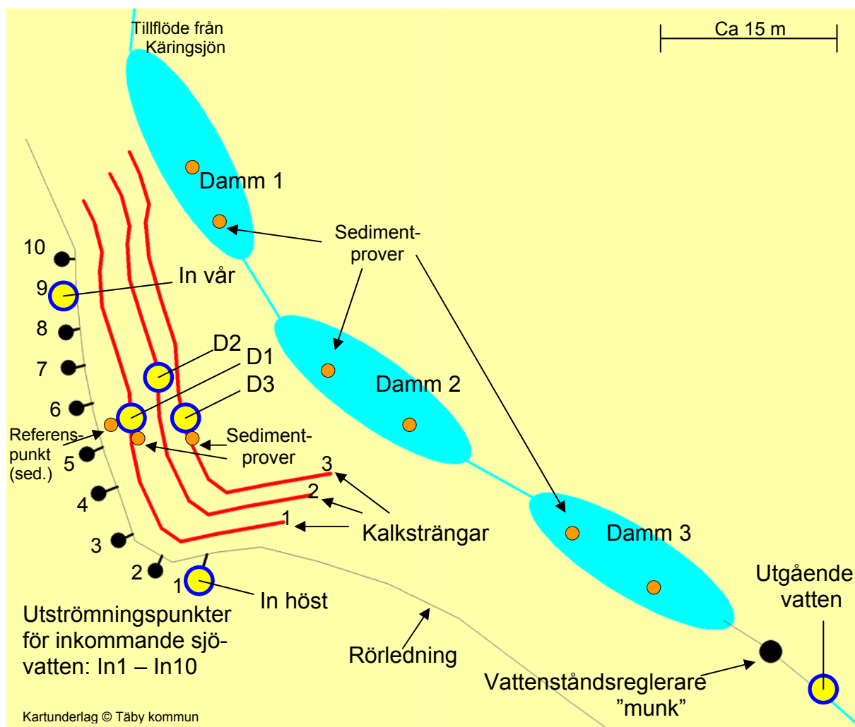
Figur nr 3. SKISS ÖVER ÖVERSILNINGSANLÄGGNING MED PROVTAGNINGSPUNKTER.
