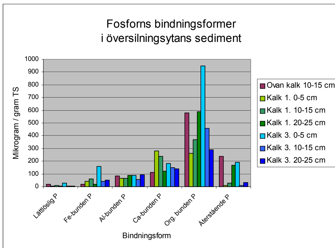
Figur nr 11: FOSFORNS BINDNINGSFORMER I ÖVERSILNINGSYTANS SEDIMENT.
