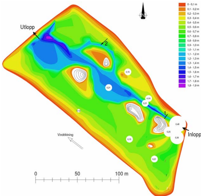
Figur 18. Jodidhalten i tio provpunkter för manuellprovtagning i Stene våtmark kl 8.00 23 april 2006. Den flödesavskärande presenningen är placerad vid 1 och behandlat hushållsavlopp mynnar i punkt 2.
