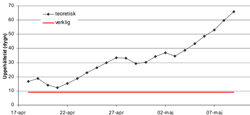
Figur 21. Den teoretiska uppehållstiden under spårämnesförsöket i våtmarken i Stene 18 april-2 maj 2006, samt verklig uppehållstid beräknad utifrån spårämnesstudien.
