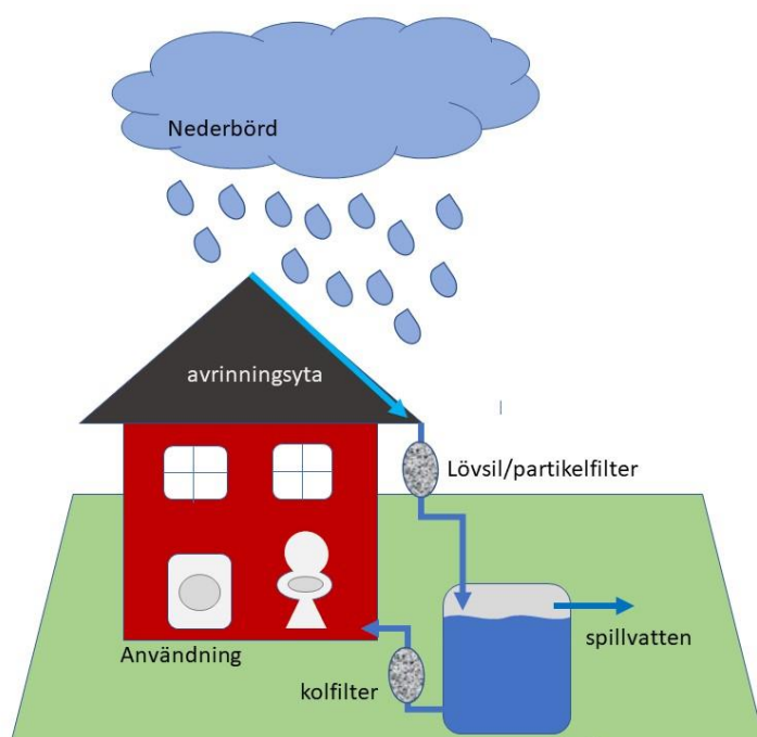
Figur 4. Huvudsakliga komponenter av ett regnvatteninsamlingssystem (egen bild).
